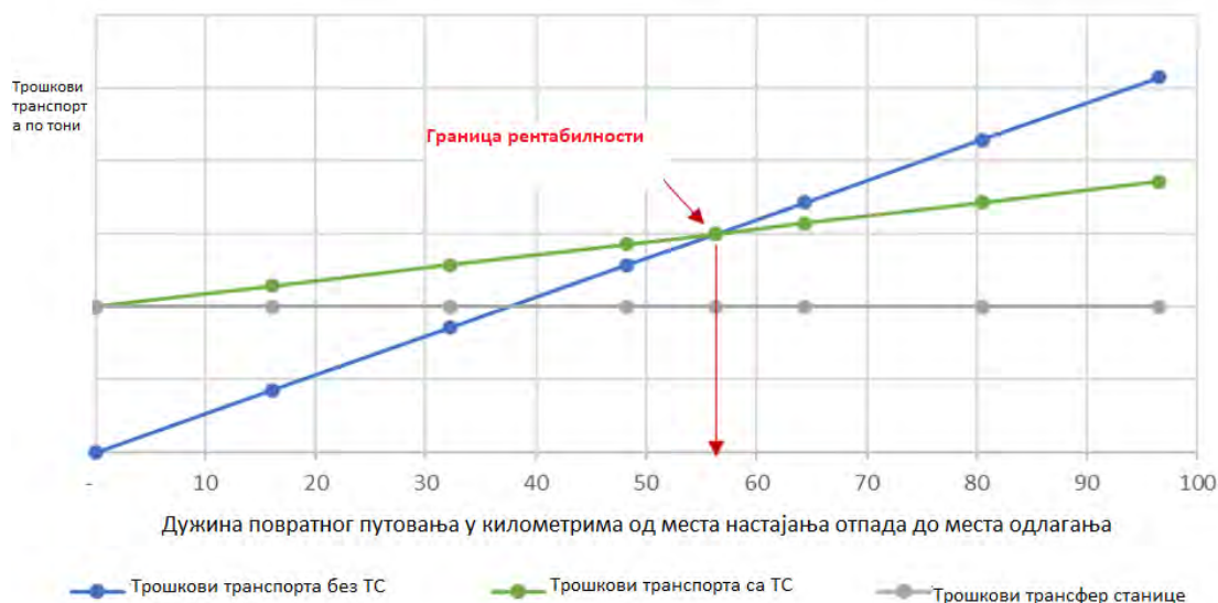
Илустрација 6-5: Пример поређења трошкова превоза са и без трансфер станице. Прилагођено из: (2002)
