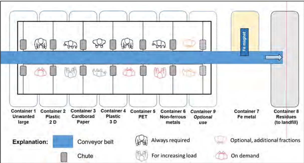
Илустрација6-14: Концепција сортирне платформе
