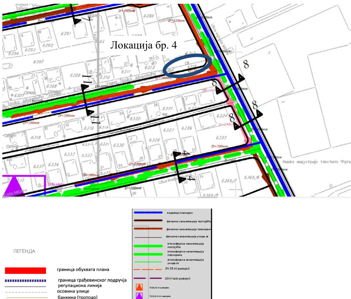
Лист бр. 7.-План инфраструктуре
